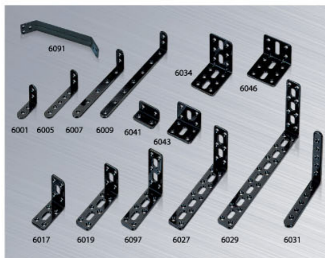
取付金具(カチオン)/L字タイプ
