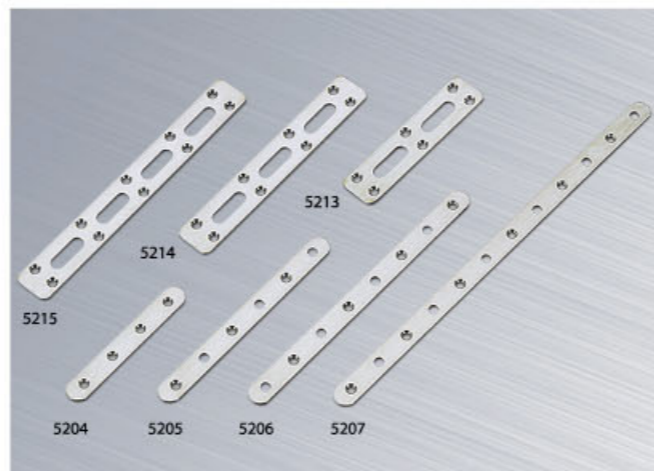
取付金具(ステンレス)/フラットタイプ
